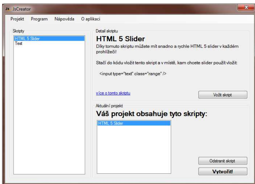
obr. 2 – rozhraní aplikace
